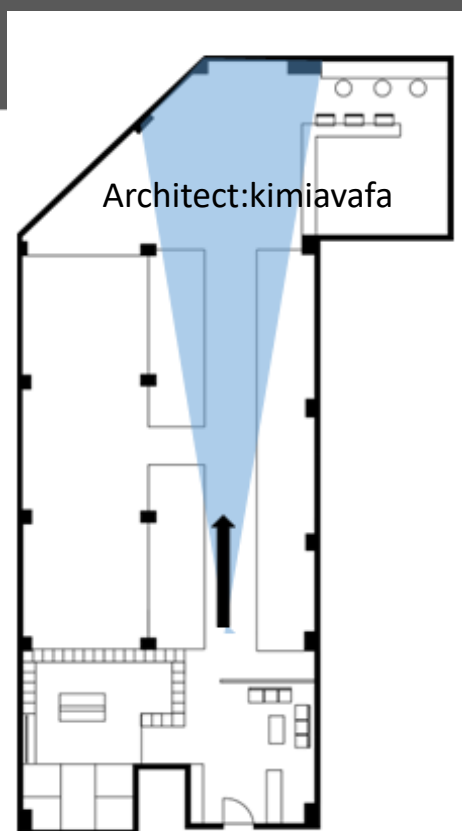
طراحی پلان
